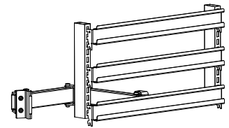
Typ 2 komplett inkl. 3 Aufhängeschienen, Länge 660 mm
