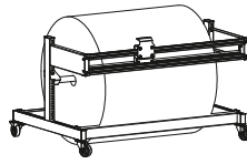
Untertisch-Schneidgerät fahrbar bis Rollendurchmesser 750 mm und 150 kg, 4 Lenkrollen Ø 125 mm, davon 2 Stk. gebremst
