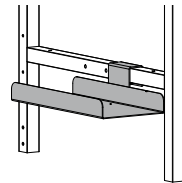
PC-Halterung zu ERGO-Basic
