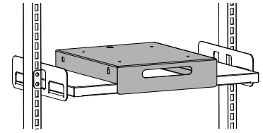
Auszugboden 100% ausziehbar für Etikettendrucker etc., Belastung max. 50 kg
