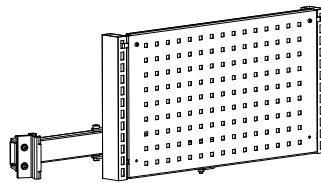
Typ 1 komplett inkl. Lochblech 660 x 370 mm
