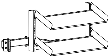
Typ 3 komplett inkl. 2 einfache Ablageböden 660 x 210 mm
