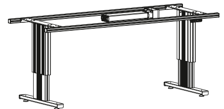
ERGO-Flex, Grundgestell mit Elektromotor höhenverstellbar mit Elektromotor von 720 – 1020 mm, Flächenbelastung 300 kg
