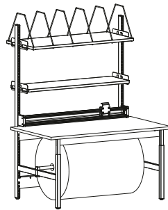
Packtisch ERGO-Budget, hoch mit Ablageboden, Faltschachtelmagazin, Rollenhalterung und Hintertisch-Schneidergerät für Rollenmaterial 125/150 cm Breite, hohe Ausführung, Flächenbelastung 200 kg
