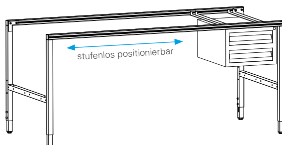
2. Schritt: Schublade
