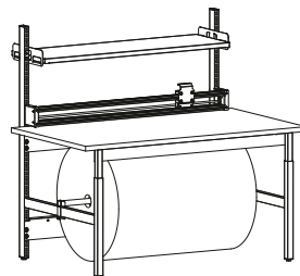
Packtisch ERGO-Budget, niedrig mit Ablageboden, Rollenhalterung und Hintertisch-Schneidergerät für Rollenmaterial 125/150 cm Breite, niedrige Ausführung, Flächenbelastung 200 kg
