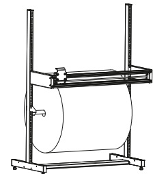
Einfach-Schneidgerät, stationär hoch für individuellen Aufbau mit Zubehör ab Seite 60, mit 1 Schneidrahmen, Achsaufnahme und Achse für Rollendurchmesser 750 mm
