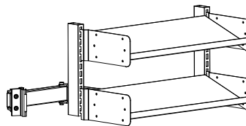
Typ 4 komplett inkl. 2 Ablageböden mit verschraubten Konsolen 660 x 270 mm
