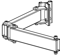
Basis zweiteilig, mit 3 Gelenken Schwenkradius 640 mm, Belastung max. 15 kg
